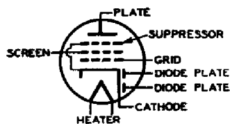
DUPLEX-DIODE PENTODE
