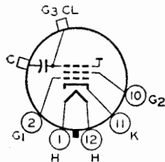
12N ULTOR = G_3 + CL
