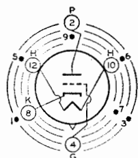
INDEX=LARGE LUG ●=PIN CUT OFF
