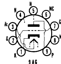
SYLVANIA TYPE 12B4 TRIODE
